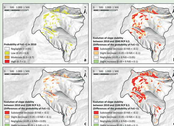
Figura 3.4.2 Evolució de la propensió a esllavissades considerant un lliscament rotacional, d'una longitud de 25m i una profunditat d'entre 1 i 3m, d'acord amb el canvi climàtic amb dos escenaris diferents: a) probabilitat mitjana d'un Factor de Seguretat (FS) ^{72} < 1 durant el període 1981-2010; b) diferències de la probabilitat d'FS < 1 entre 1981-2010 i 2040 amb escenaris RCP 4.5; c) diferències en la probabilitat d'FS < 1 entre 1981-2010 i 2100 amb escenaris RCP 4.5; d) diferències de la probabilitat d'FS < 1 entre 1981-2010 i 2100 amb escenaris RCP 8.5. Font: Projecte SAMCO, 2018.
