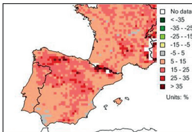
Figura 3.2.6. Estimació de la diferència del creixement relatiu (en %) de M. phaseolina l'any 2030 respecte a les condicions climàtiques del 2012. El color vermell fosc indica l'increment màxim del creixement relatiu. Font: Manigi et al., 2012.
