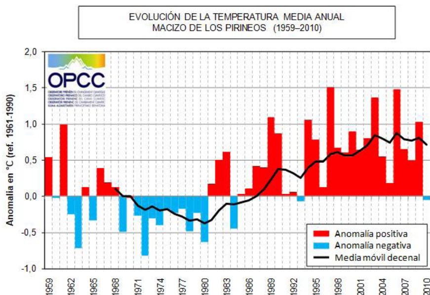
Figura 1.2.1 Evolució de la temperatura mitjana anual al conjunt dels Pirineus durant el període 1959-2010. Es mostra l'anomalia anual respecte del valor mitjà del període referència 1961-1990 (línia vermella: positiva; línia blava: negativa) i l'evolució de la mitjana mòbil per a un període de 10 anys (línia negra). Font: OPCC, 2013
