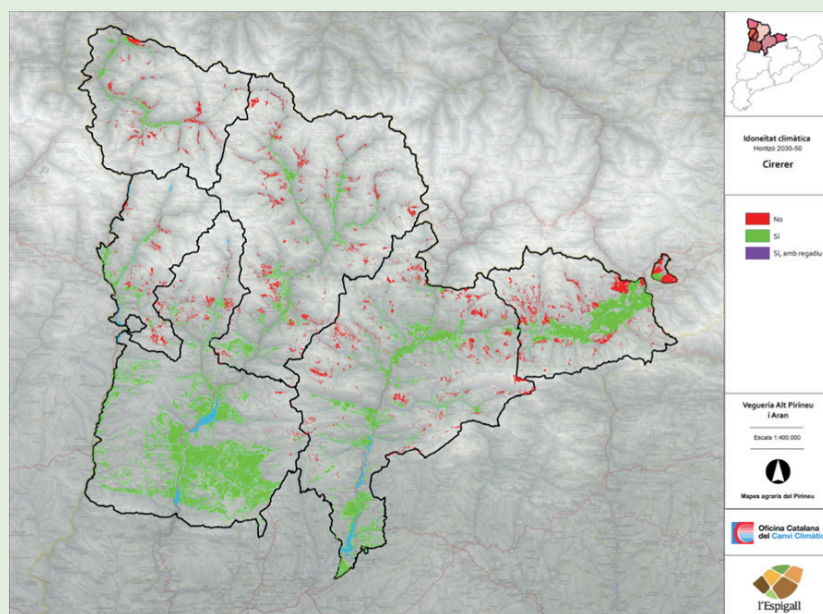
Figura 3.2.5. Mapa de idoneïtat climàtica projectada per al cultiu del cerezo en el Alto Pirineo y Arán para el periodo 2030-50, respecto a la idoneïtat climàtica actual.
