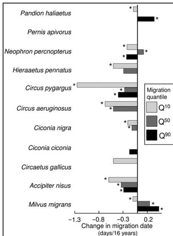
Figura 2.2.1. Estimació de l'avançament de la data d'arribada a la Península Ibèrica d'11 espècies d'aus migratòries entre els anys 1999 i 2011 (dies corresponents a 16 anys). El color gris clar representa el Q10 i correspon al 10 % de les aus comptades. El color gris fosc representa el Q50 i correspon al 50 % de les aus comptades i el color representa el Q90 i representa el 90 % de les aus comptades. Font: Panuccio et al., 2017
