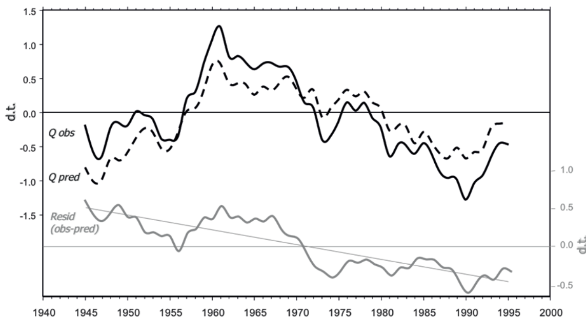
Figura 2.6.2. Evolució de les aportacions anuals dels rius dels Pirineus centrals espanyols ( Q_{obs} ) i dels cabals teòrics a partir només de les dades climàtiques ( Q_{pred} ). El residual o diferència entre cabals predits i observats (Resid) mostra una evolució descendent dels cabals que no queda explicada per la variabilitat climàtica, i que s'atribueix a l'increment de l'evapotranspiració a causa dels canvis d'ús i de vegetació. Font: adaptat de Beguería et al., 2003.
