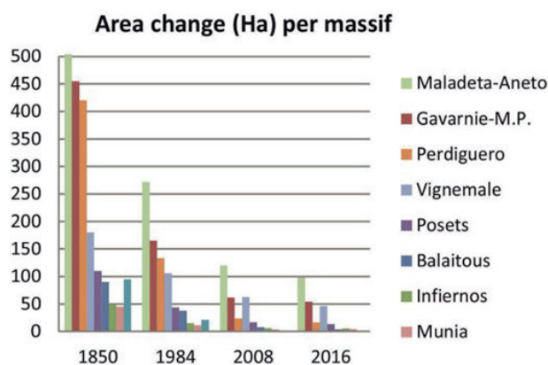
Figura 3.1.4. Estimació de l'evolució de l'àrea dels principals massissos glaciers dels Pirineus. Font: Rico et al., 2017
