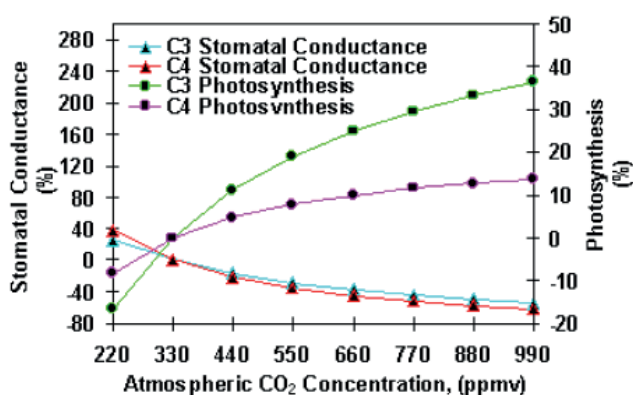
Figura 3.2.4. Corba d'increment de l'eficiència fotosintètica i disminució de la conductància estomàtica a les plantes amb un metabolisme C3 i C4, en funció de la concentració de CO 2 a l'aire. Font: AVEMAC project; JRC., 2012
