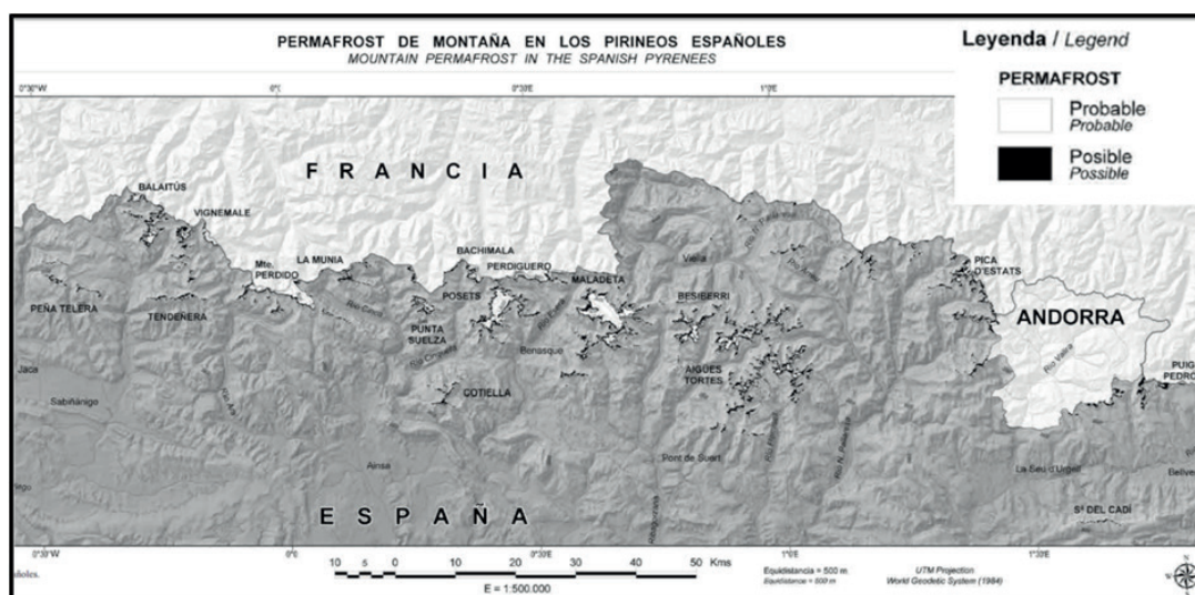
Figura 3.4.3. Presència, possible i probable, de pergelisol als Pirineus espanyols (modificat de Serrano et al., 2009).
