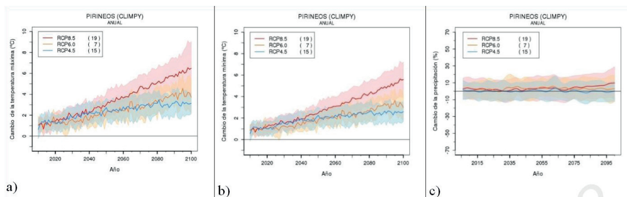
Figura 1.3.1 Evolució de l'anomalia mitjana anual de la (a) temperatura màxima, (b) temperatura mínima i (c) precipitació mitjana als Pirineus. Font: projecte CLIMPY.
