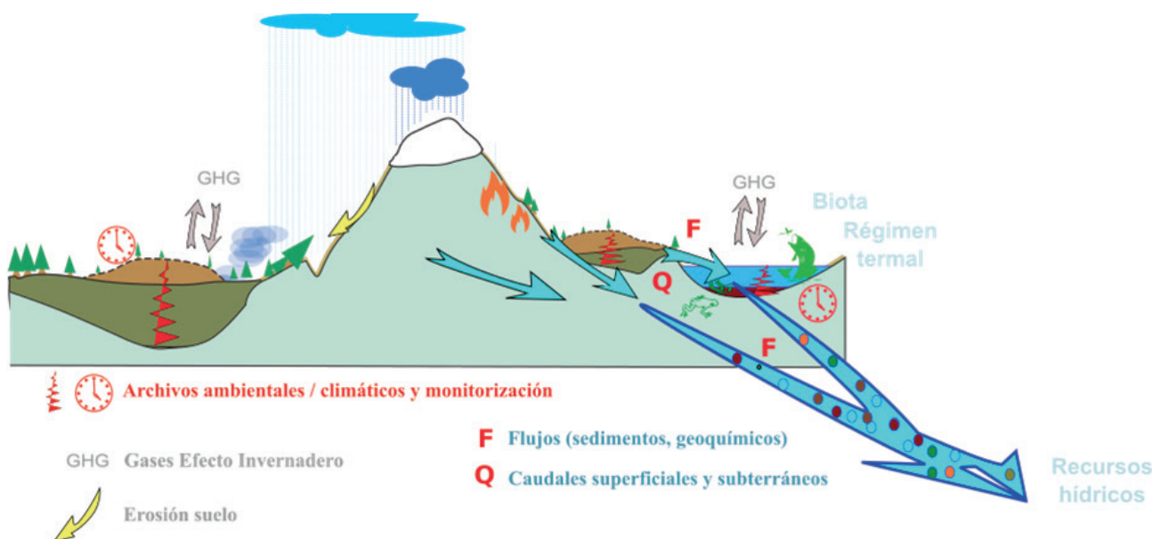
Figura 2.5.1. Cicles biogeoquímics en els estanys i torberes d'alta muntanya. Font: Projecte REPLIM
