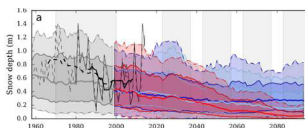
Figura 1.3.2 Evolució de la distribució estadística del gruix mitjà de neu als Pirineus centrals (altitud 1.800 m) a partir de la sèrie de l'observatori de La Mongie (línia negra contínua), les simulacions històriques (línia gris) i de la reanàlisi Safran (línia negra puntejada) per al futur del conjunt EURO-CORDEX amb les RCP 2.6 (blau fosc), RCP 4.5 (blau clar) i RCP 8.5 (vermell). Font: Météo-France
